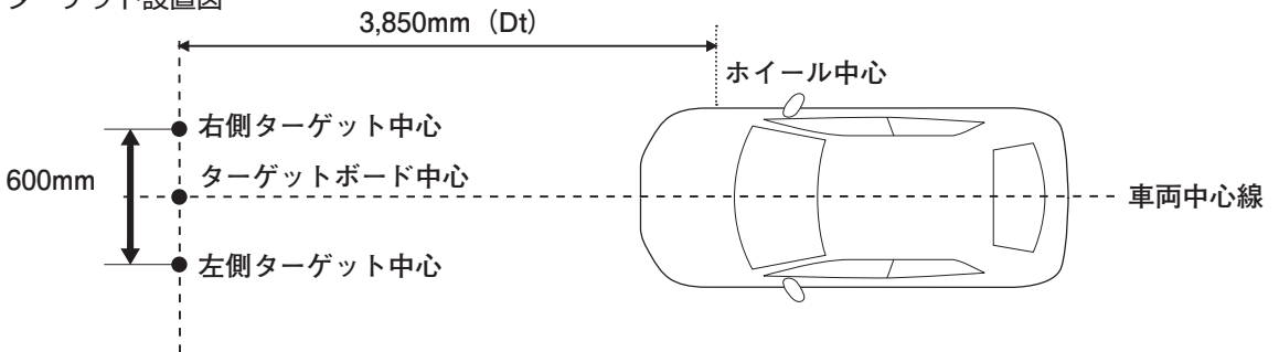
ターゲット設置図
