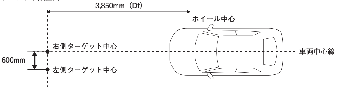
ターゲット設置図
